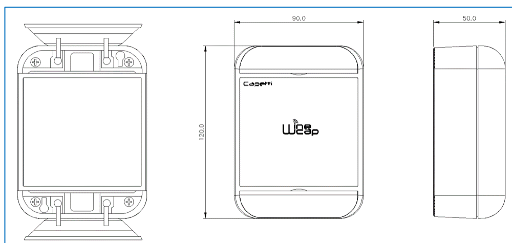
Figura 8 - Dimensioni meccaniche
