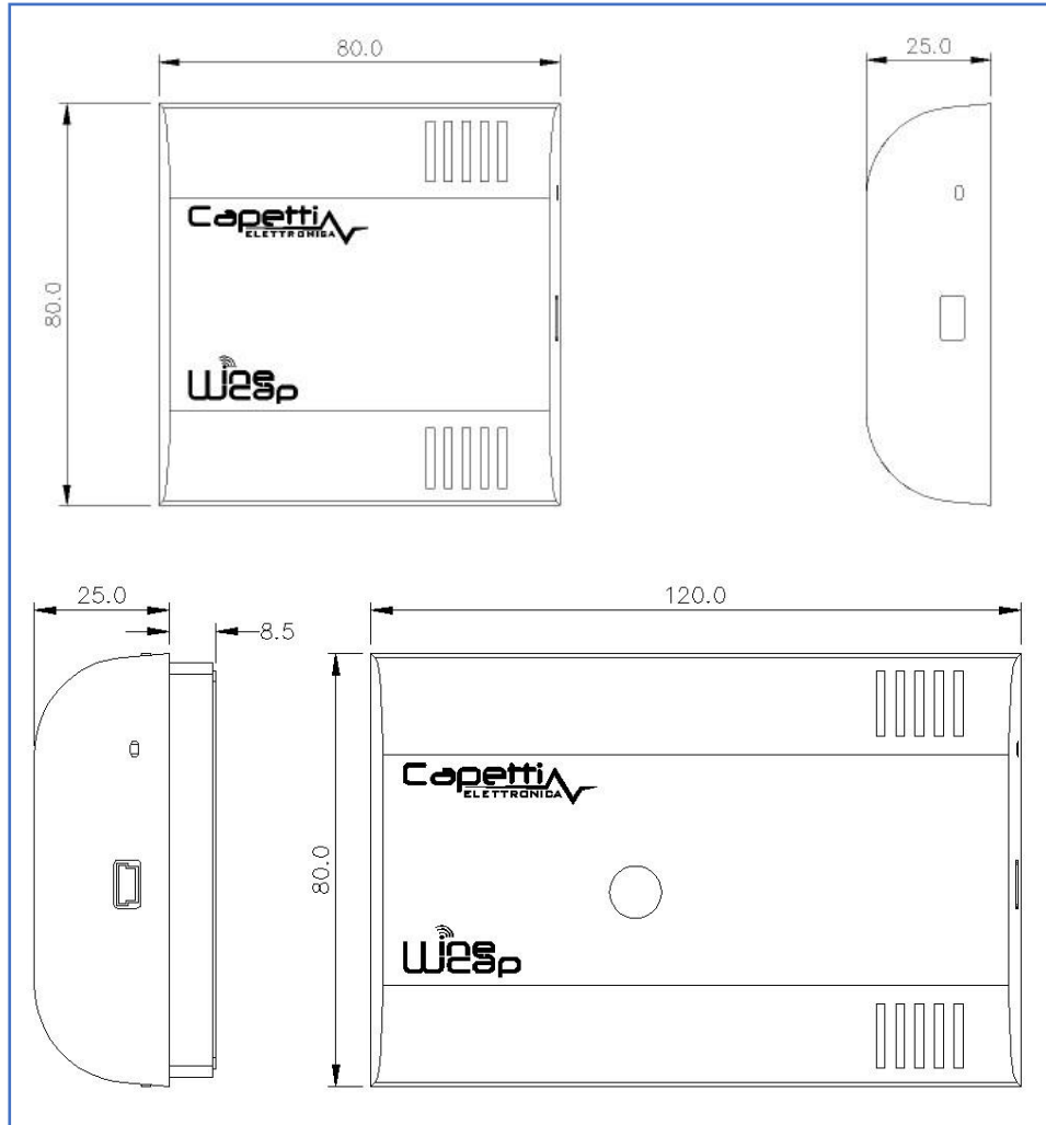
Figura 7 - Dimensioni meccaniche
