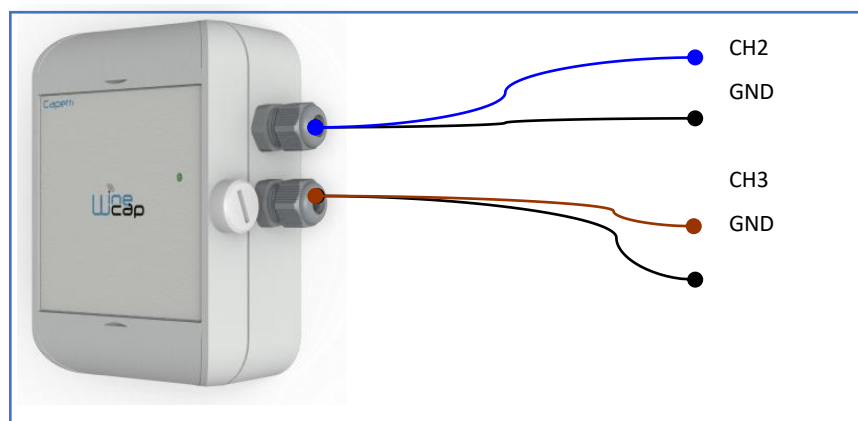
Figura 7 - Layout collegamenti
