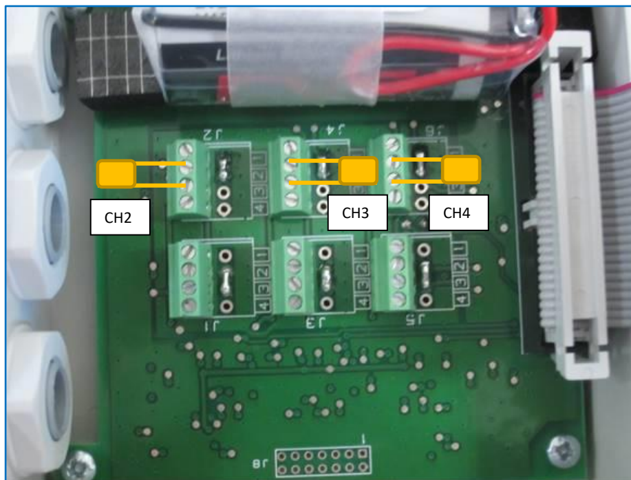
Figura 7 - Layout collegamenti
