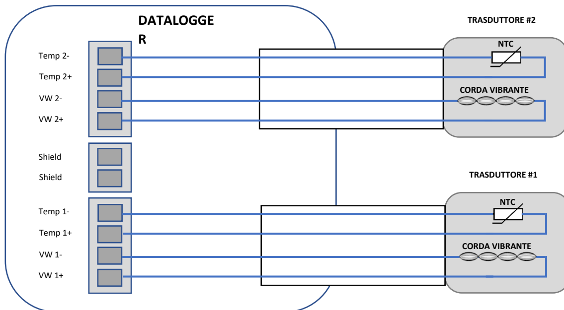
Figura 6 - Layout collegamenti
