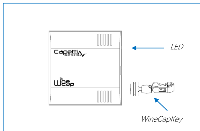
Figura 3 - Posizionamento WineCapKey
