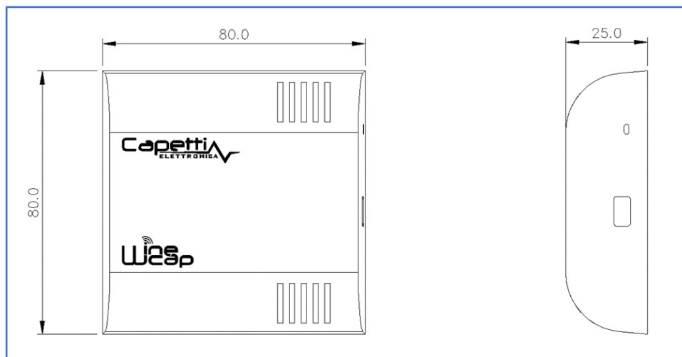
Figura 7 - Dimensioni meccaniche
